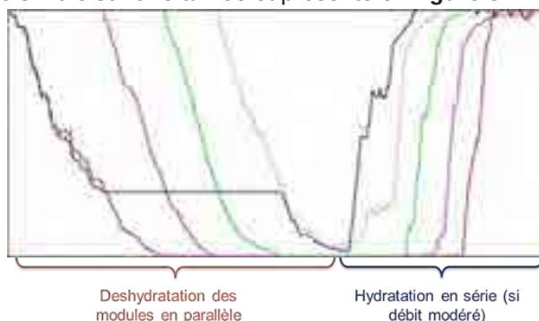
Figure 3 : Gestion de la charge et de la décharge d'un ensemble de 5 réacteurs simulés dans un système complet
