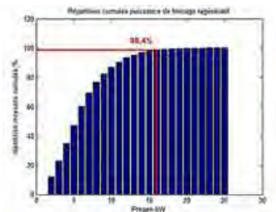
Figure 1 : Répartition cumulée de l'énergie de freinage en fonction de la puissance de freinage (moyenne sur cinq cycles)
