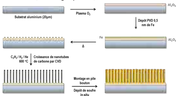
Figure 3 : Procédure de croissance des tapis de nanotubes de carbone. Le substrat de départ est un feuillard d'aluminium couramment utilisé comme collecteur de courant dans les batteries. Après la croissance, l'électrode est introduite dans un accumulateur, et le soufre est déposé lors de la charge
