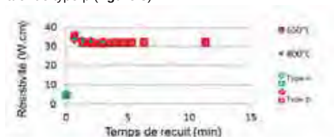
Figure 8 : Résistivité en fonction du temps de recuit de destruction de donneurs thermiques
