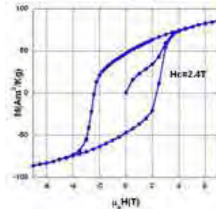
Figure 4 : Courbe M(H) mesurée à température ambiante après co-broyage de 12h d'un mélange NdFeB+30wt%Nd 70 Cu 30 et recuit à 520°C, 1h.
