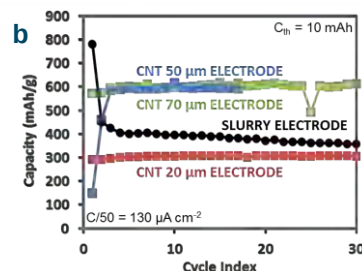
Figure 5b : Courbes de cyclage de différents accumulateurs Li/S : avec électrode composite (noir), avec des NTC sur aluminium de différentes hauteurs \rightarrow 20 \mu\text{m} (rouge), 50 \mu\text{m} (bleu) et 70 \mu\text{m} (vert)
