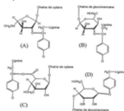
Figure 2 : Exemples de liaisons LCC des lignines issues de bois intact et préhydrolysé
