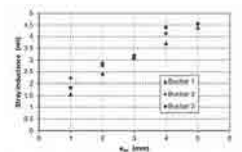
Figure 2b : Résultats des mesure directes d'inductance
