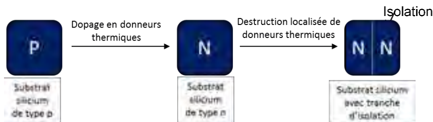
Figure 3 : Schéma de principe de la réalisation de l'isolation des cellules haute tension
