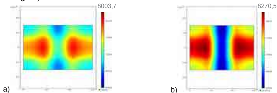
Figure 4 : Vue de dessus de la modélisation de la densité de courant produite (en A/m²) pour des gaz hydratés à la cathode (A) à 25% et (B) à 75% d'humidité relative. Le canal cathodique est vertical, le canal anodique est horizontal.
