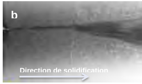
Figure 4b : Topographie X en faisceau blanc en coupe longitudinale
