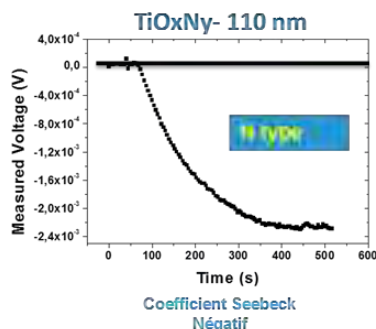
Figure 6. Détermination du type de conduction par mesures Seebeck.
