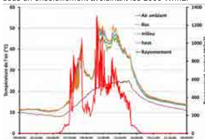
Figure 12 : Évolution des température d'air au sein du prototype pour une journée de fin d'été
