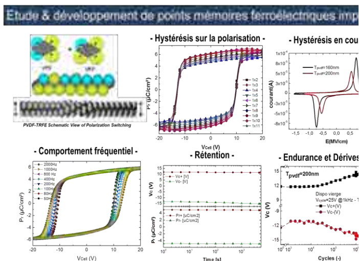
Figure 1 : illustration des caractéristiques de la technologie Mémoire Non-Volatile développée au Liten
