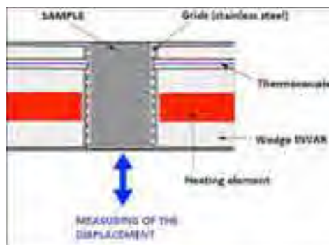
Figure 2 : Schéma du porte-échantillon
