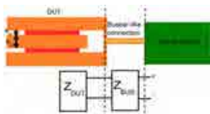
Figure 2a : Principe de mesure directes d'inductance
