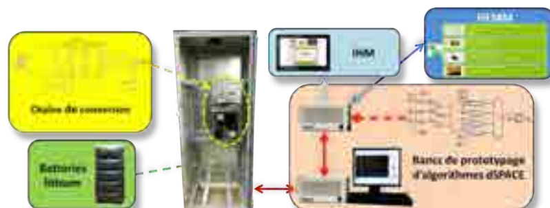
Figure 3 : Schéma de principe de la maquette de systèmes d'autoconsommation
