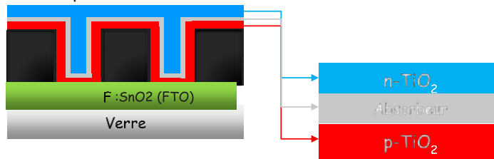
Figure 1 : Hétérostructure à base de \text{TiO}_2 , envisagée pour la fabrication d'une cellule solaire (ou d'une jonction p/n sans la couche absorbeur).
