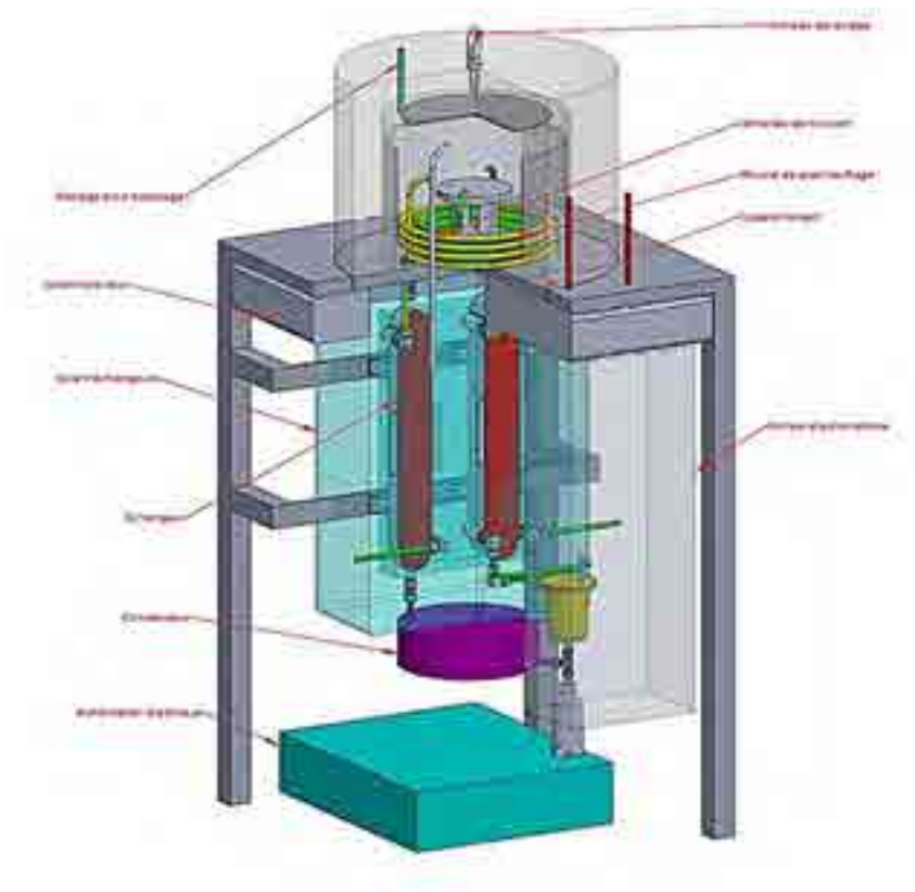
Figure 3 : schéma 3D de l'installation
