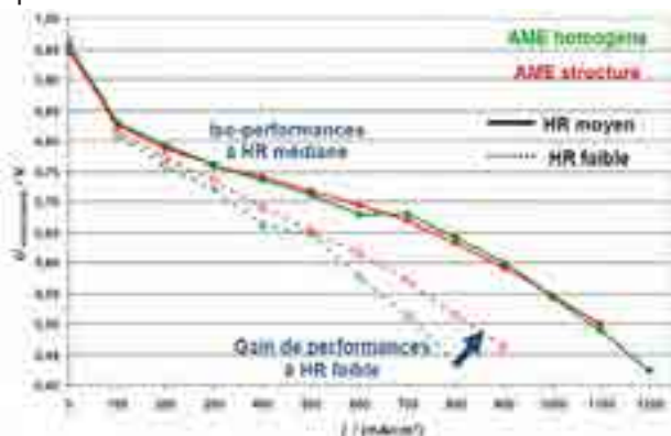
Figure 2 : Comparaison des performances entre un AME 220 cm 2 homogène et structuré en fonction des conditions d'humidité des gaz
