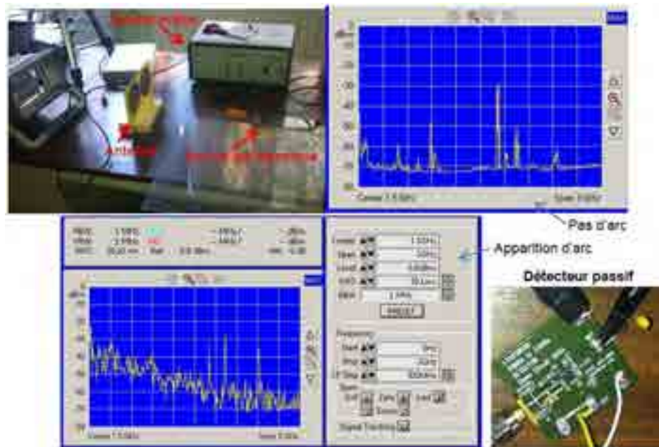
Figure 2 : Détection de la source d'arc électrique à travers la signature électromagnétique Ainsi la détection électromagnétique constitue le premier niveau de traitement et qui, effectuée à l'aide des dispositifs passifs, offre l'avantage de l'autonomie du système. Une fois la signature électromagnétique détectée, le deuxième niveau de traitement est déclenché, celui basé sur la localisation à l'aide de l'antenne ultrasonore illustrée sur la figure 3 .
