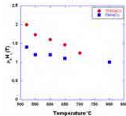
Figure 5 : Coercivité en fonction de la température de recuit des poudres obtenues par cobroyage (3 heures) de NdFeB avec respectivement 5% ou 30% d'alliage Nd 70 Cu 30 .
