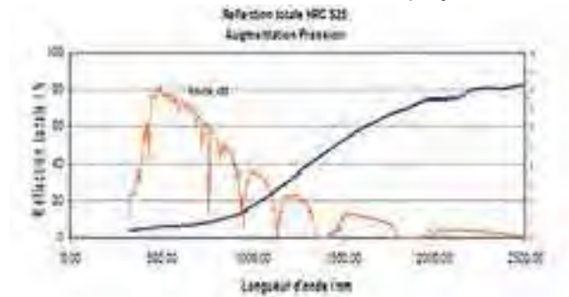
Figure 2 : Réflectivité de couches métalliques structurées présentant une forte absorption dans le domaine visible du rayonnement solaire
